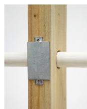
Protección de cable con la placa NS fijada sobre cabrios de madera
