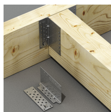
Fijación viga/viga
