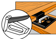
Fijación del CLIP con grapa
